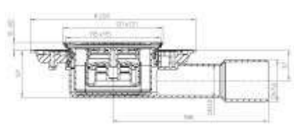
Рис. 2. Трап HL90.Prblue-3000
