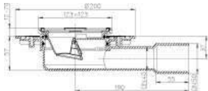
Рис. 1. Трап HL90.2
