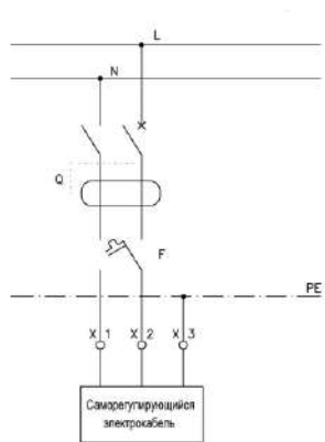
Рис. 2. Схема подключения
