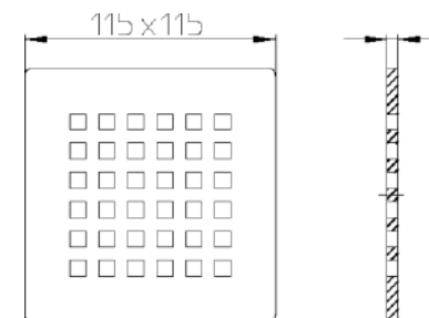
Рис. 3. Декоративная решетка HL3120 (Quadra).
