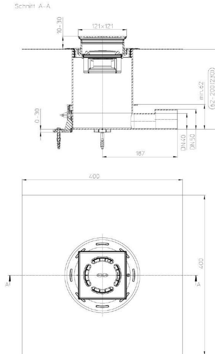
Рис. 1. Трап HL541.
