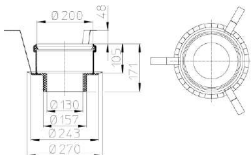
Рис. 2. Противопожарная муфта HL860 для трапа HL616/1.
