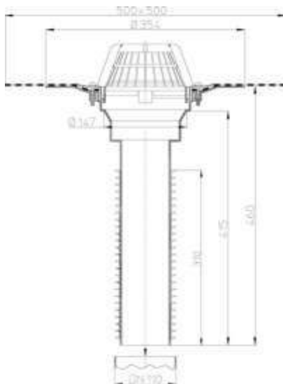
Рис. 2. Кровельная воронка HL69H/1.
