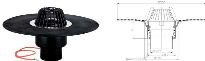
Рис. 3. Кровельная воронка с электрообогревом для внутреннего водостока HL62.1H/2.
