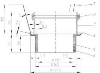
Рис. 6. Противопожарная муфта HL870 для кровельной воронки HL62.1H/1.
