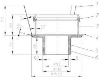
Рис. 5. Противопожарная муфта HL850 для кровельной воронки HL62.1H/7.
