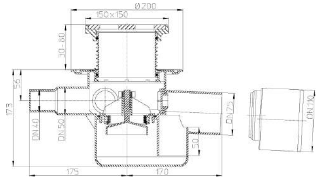
Рис.1. Трап HL70G
