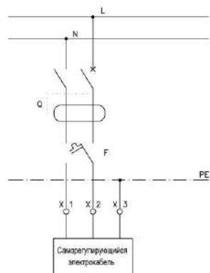
Рис. 4. Схема подключения электрообогрева кровельной воронки HL63.1Н к электрической сети.
