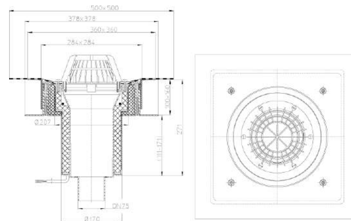
Рис. 1. Кровельная воронка HL63.1H/7.
