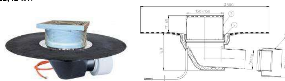
Рис. 1. Кровельная воронка с электрообогревом HL64.1BH
