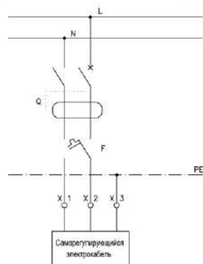
Рис. 2. Схема подключения электрообогрева кровельной воронки HL64.1BH к электрической сети.
