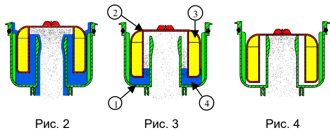
Рис.2. Сифон во время слива воды. Рис.3. Пересыхание водяного затвора. Рис.4. Сифон в «сухом» состоянии.
