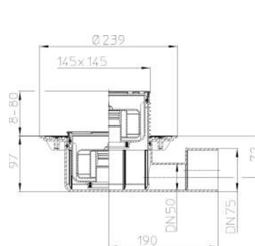
Трап HL5100Pr
